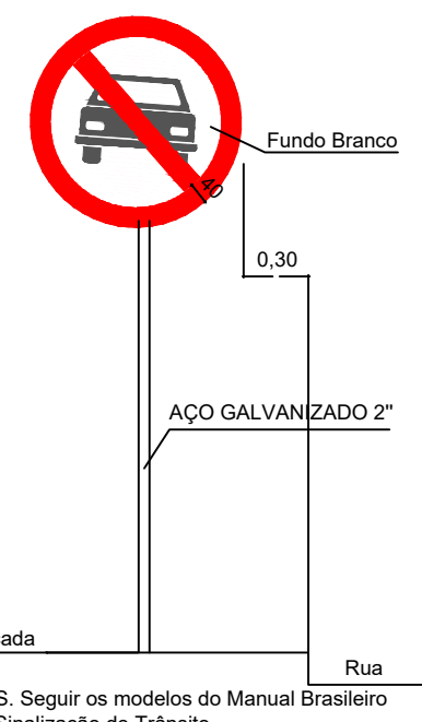
DETALHE PLACA Proibido trânsito de veículos automotores R-10
