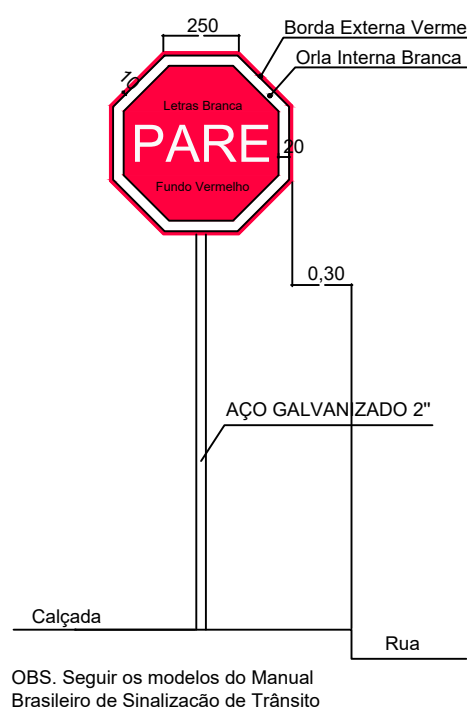
DETALHE PLACA PARE - R-1
