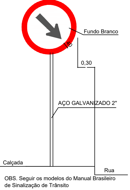
DETALHE PLACA Passagem obrigatória R-24b (40 km/h)
