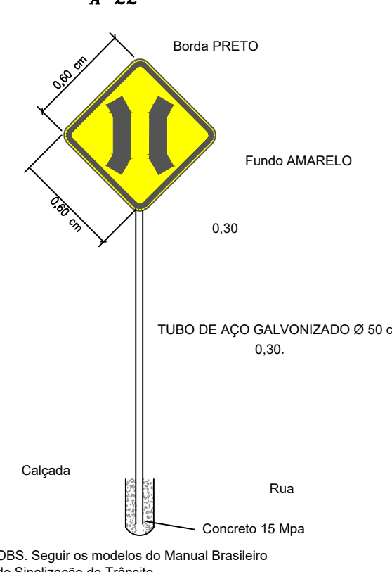
DETALHE PLACA DE PONTE ESTREITA A-22
