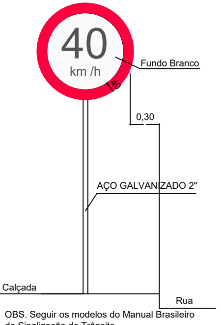
DETALHE PLACA VELOCIDADE MÁXIMA R-19 (40 km/h)
