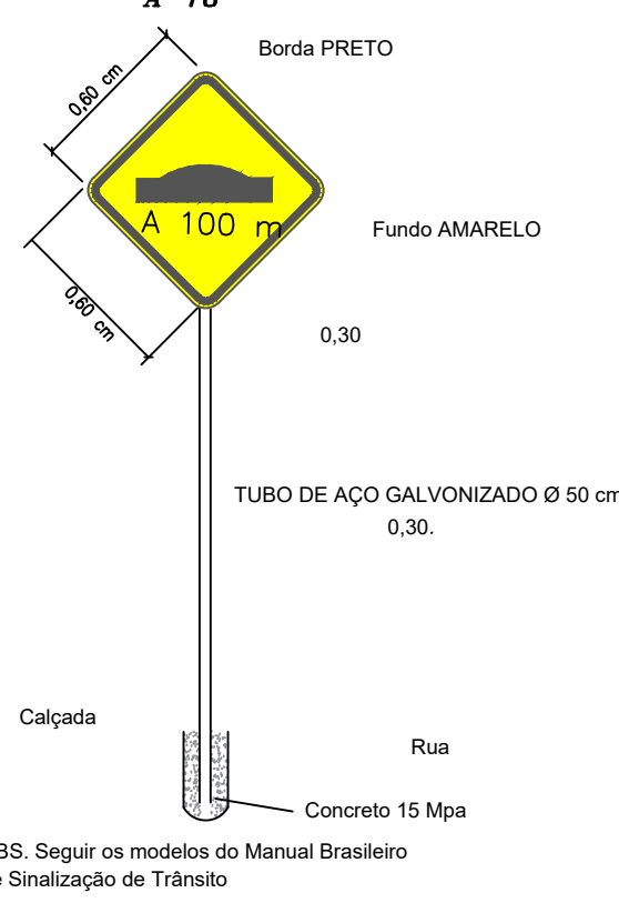
DETALHE PLACA DE SALIÊNCIA OU LOMBADA A-18
