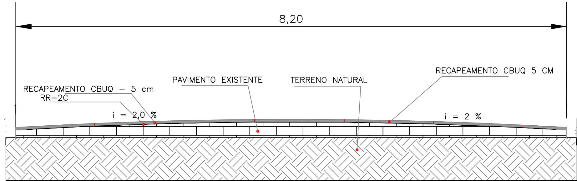
PERFIL TRANSVERSAL SEM ESCALA
