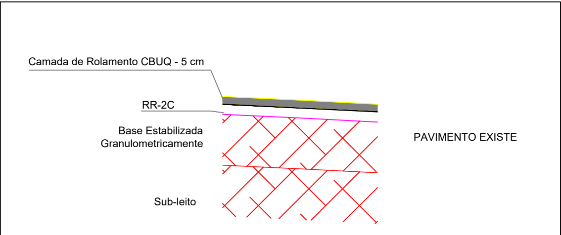
DETALHAMENTO – ESPESSURA DO PAVIMENTO S/ ESCALA
