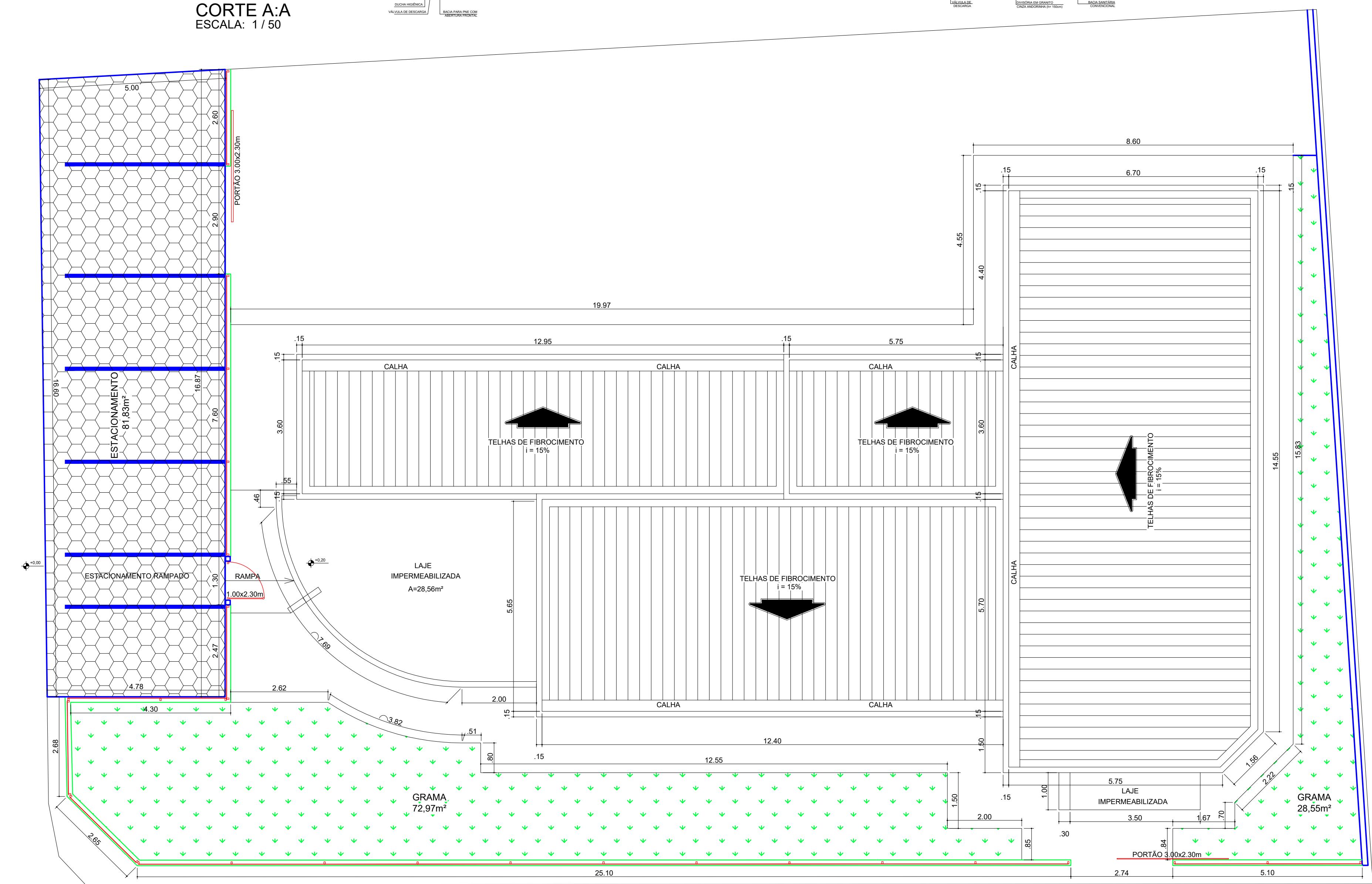
PLANTA DE LOCAÇÃO/COBERTURA/ACESSIBILIDADE ESCALA: 1 / 75
