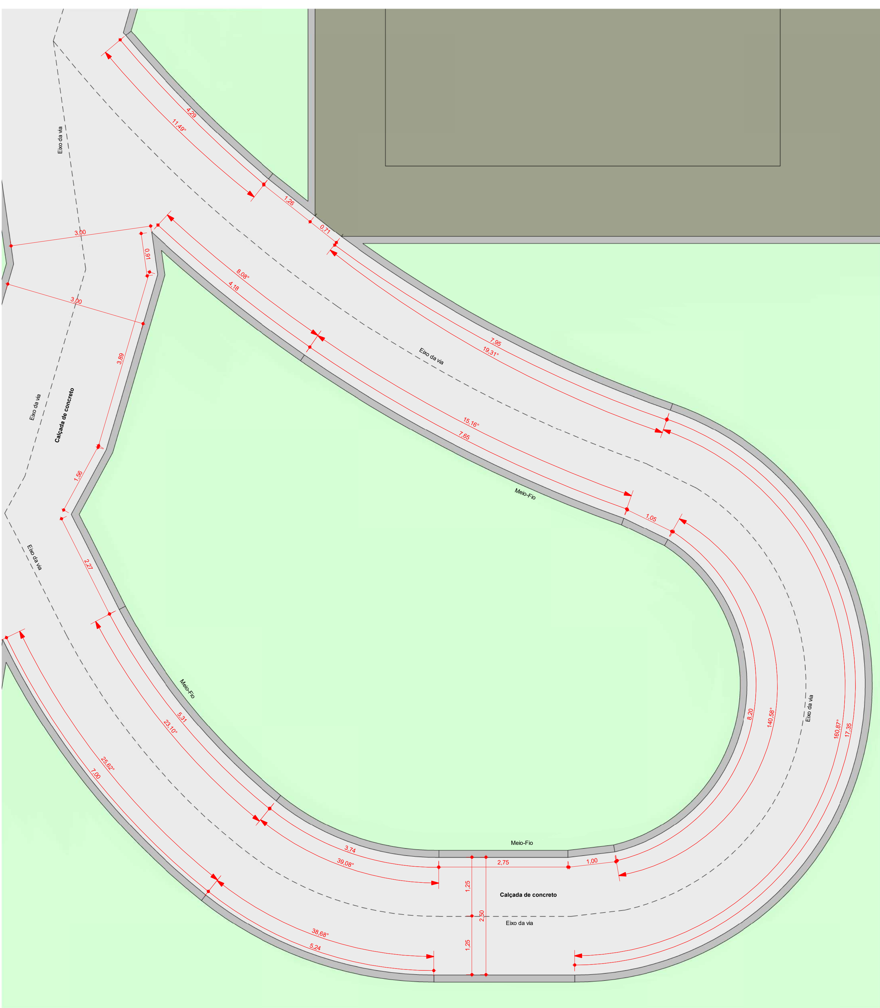
3 Trecho 07 ESCALA - 1 : 50
