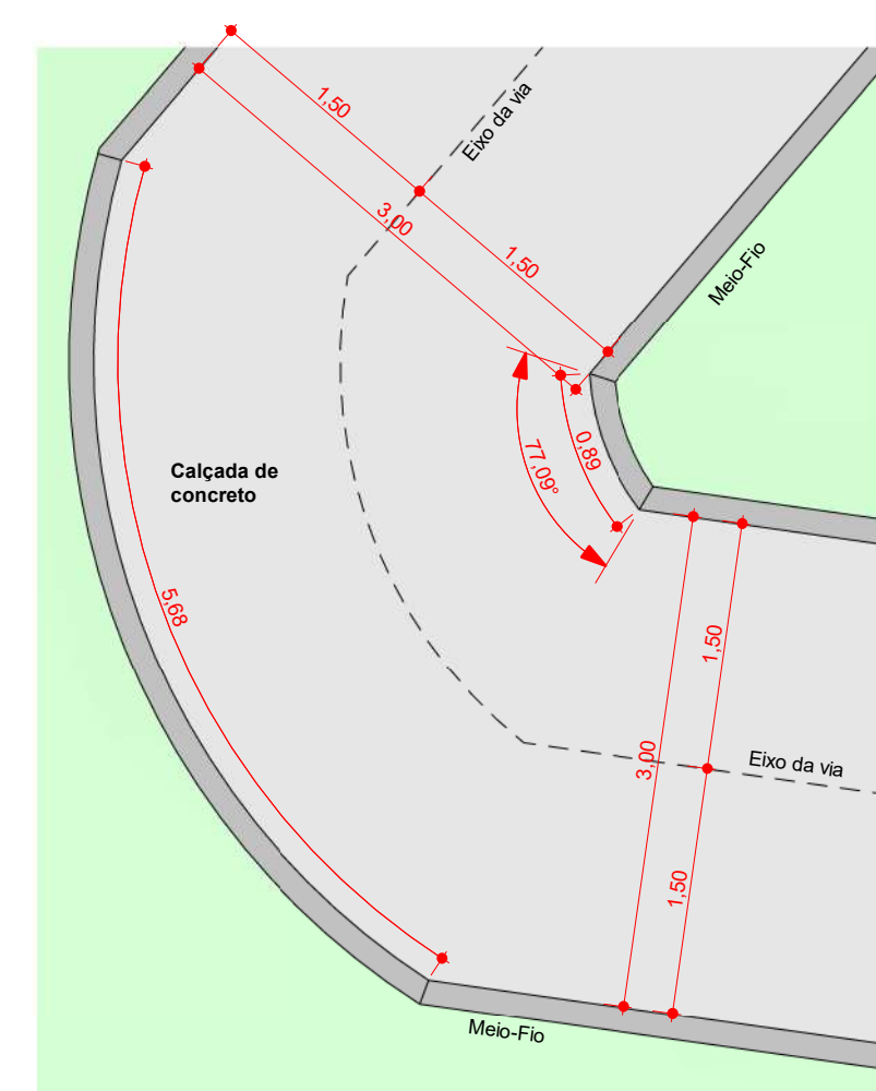
11 Trecho 09 ESCALA - 1 : 50
