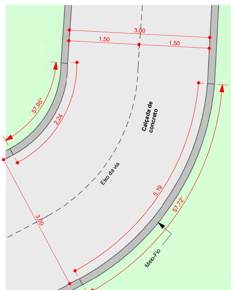
10 Trecho 08 ESCALA - 1 : 50
