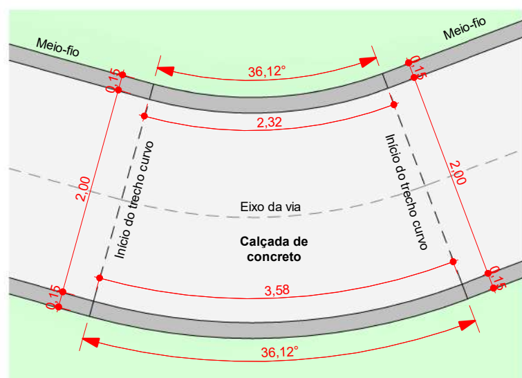
7 Trecho 04 ESCALA - 1 : 50
