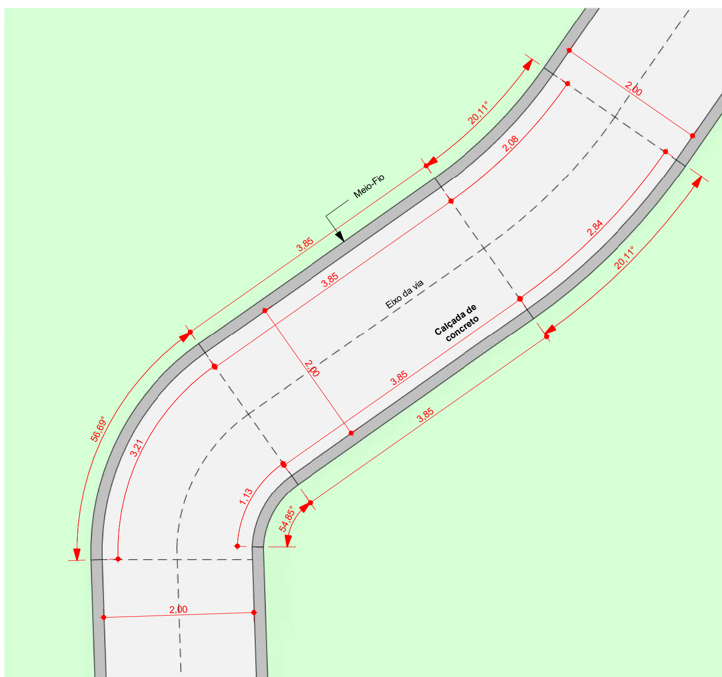
5 Trecho 02 ESCALA - 1 : 50
