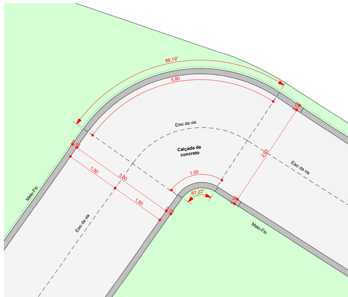
4 Trecho 01 ESCALA - 1 : 50
