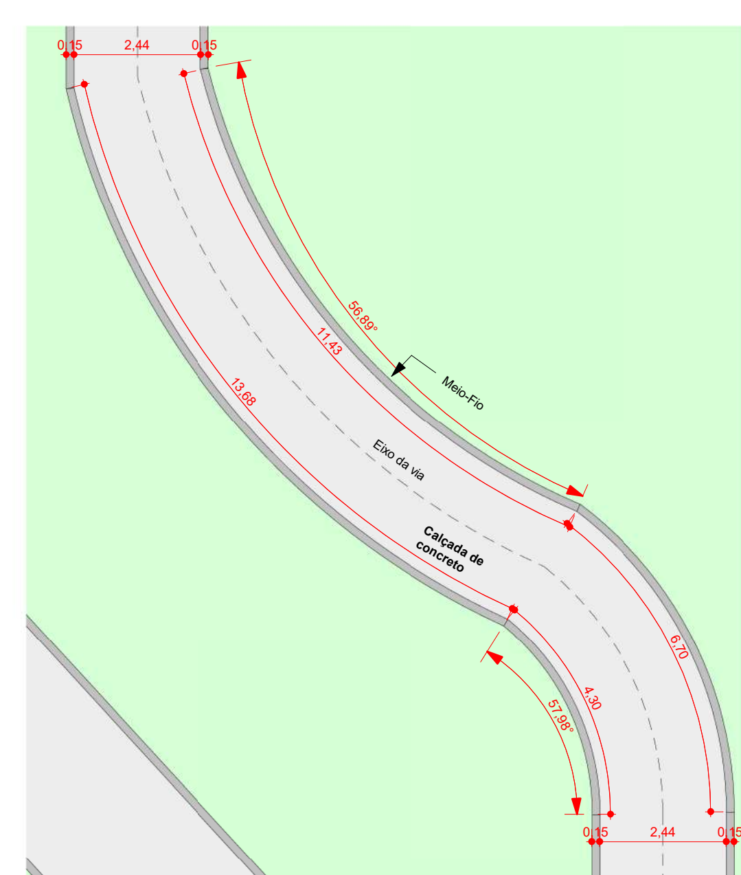
12 Trecho 10 ESCALA - 1 : 100
