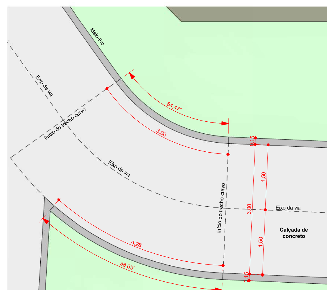
9 Trecho 06 ESCALA - 1 : 50
