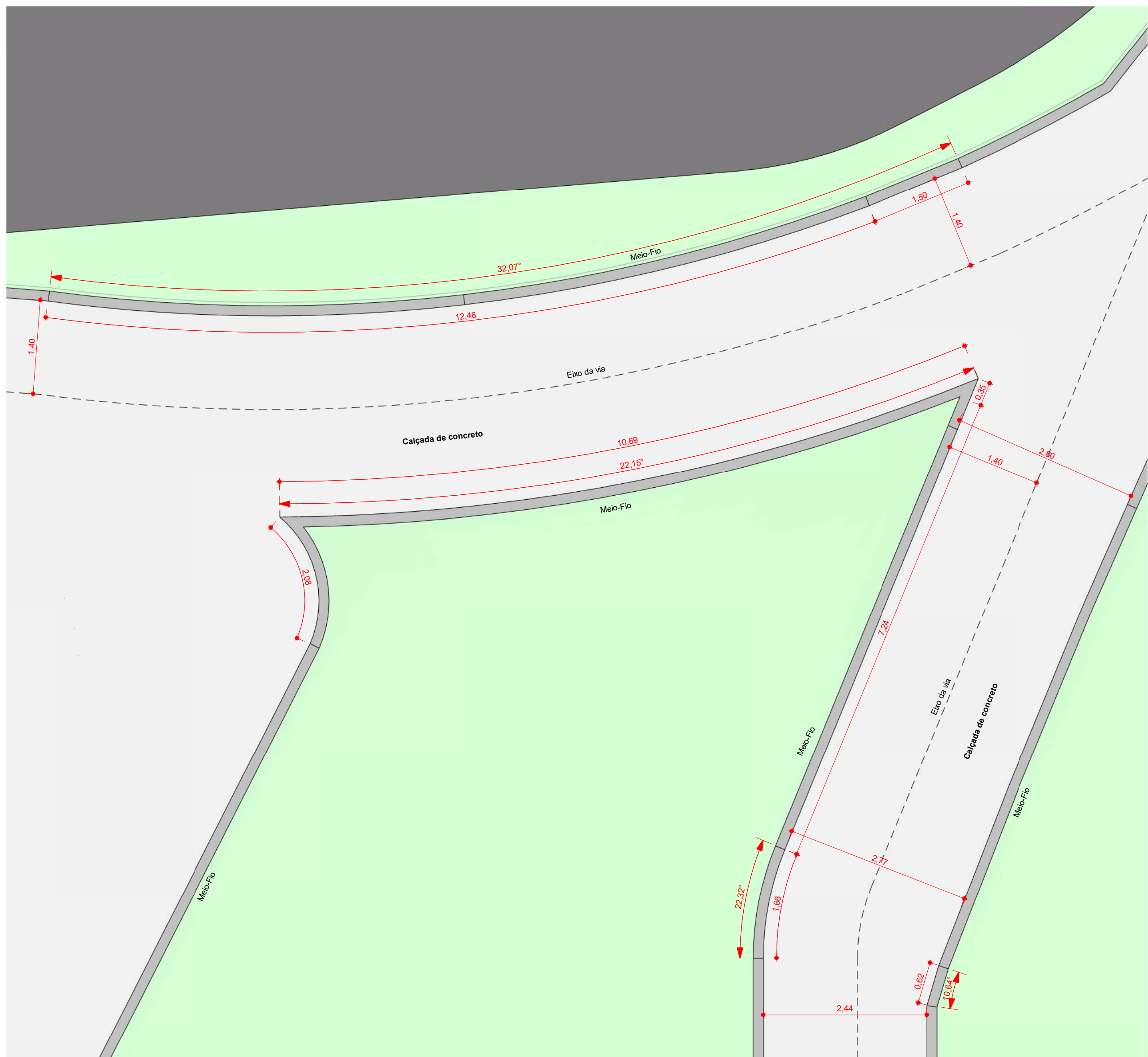
2 Trecho 13 ESCALA - 1 : 50
