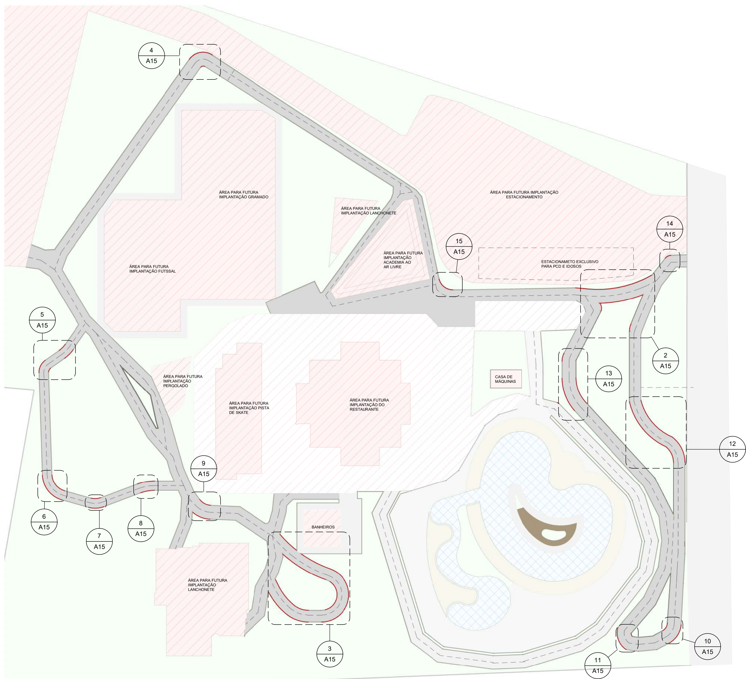
1 Pista de cooper - Planta Chave ESCALA - 1 : 500
