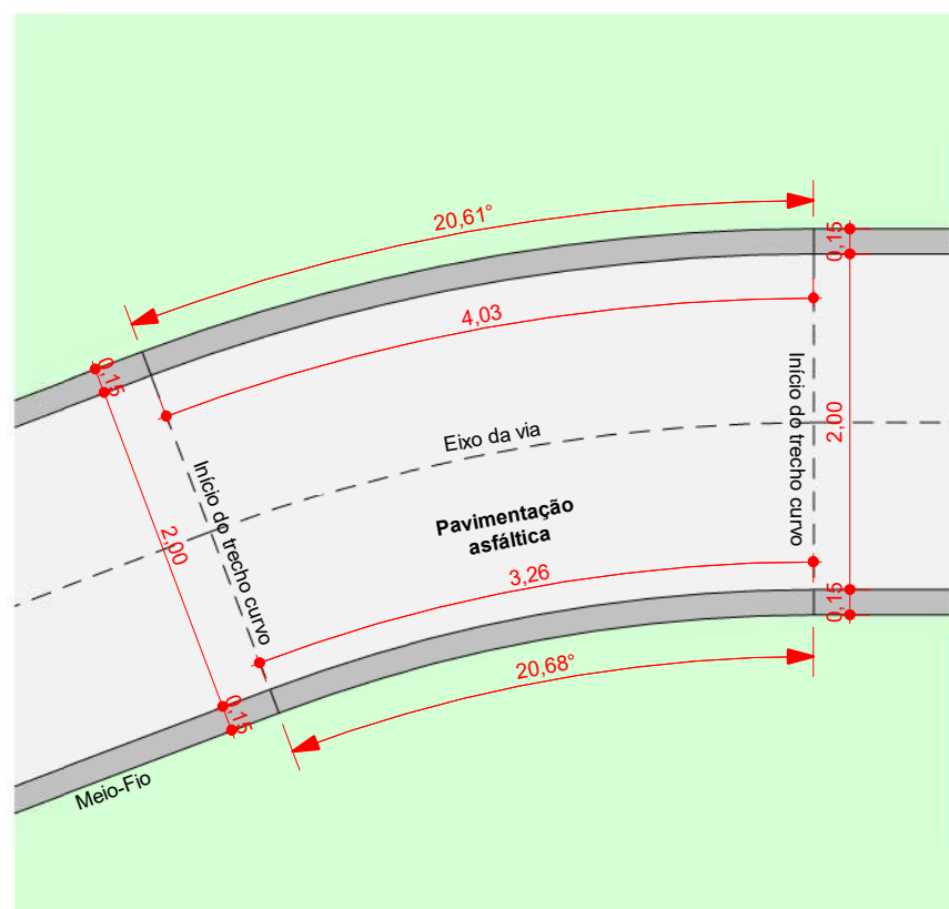
8 Trecho 05 ESCALA - 1 : 50
