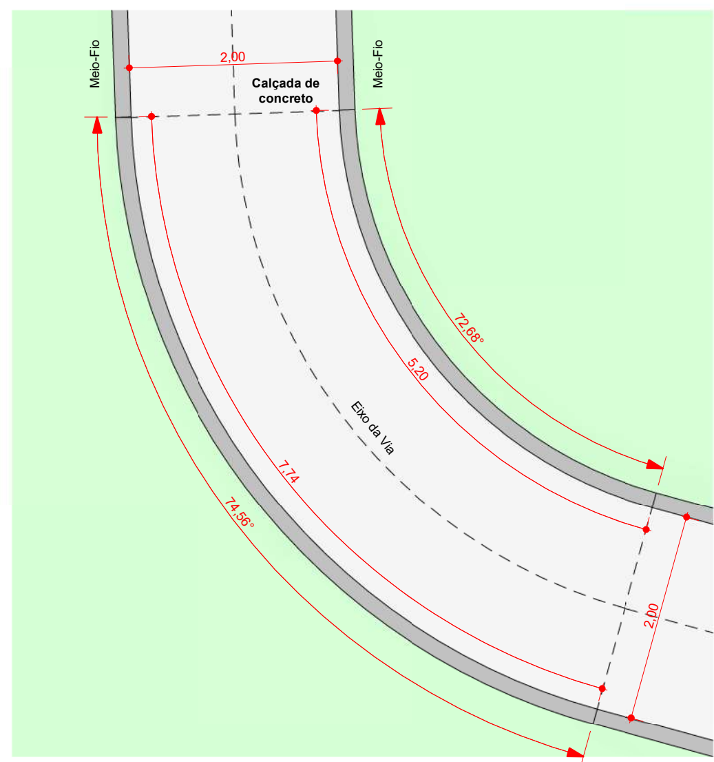
6 Trecho 03 ESCALA - 1 : 50
