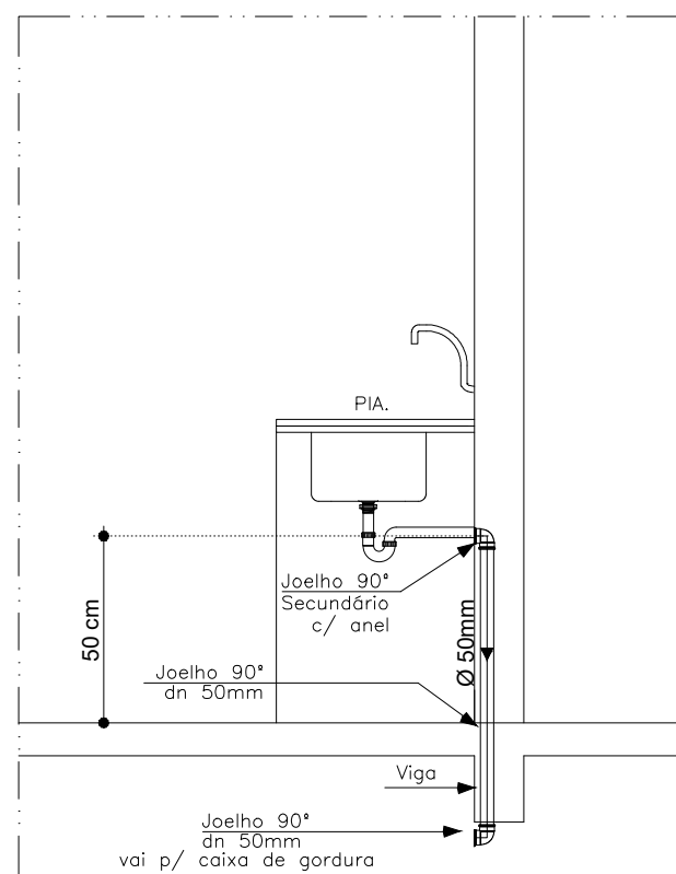
DETALHE PIA ESC: 1/25
