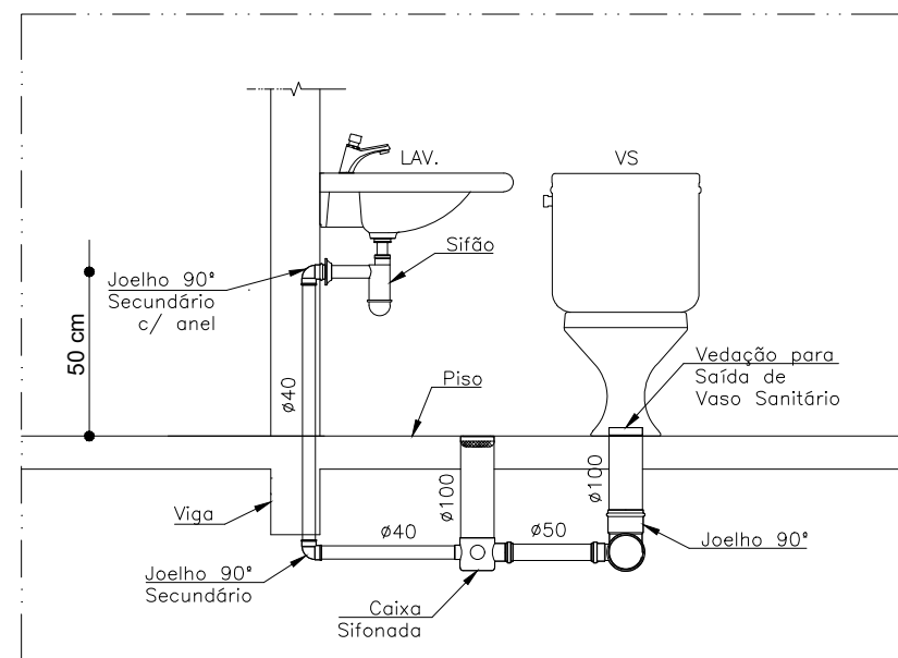
DETALHE SANITÁRIO ESC: 1/25
