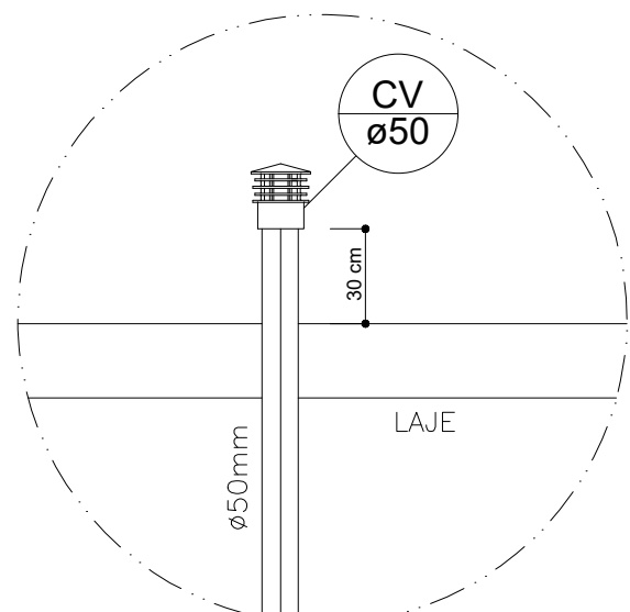
DETALHE COLUNA DE VENTILAÇÃO SEM ESCALA
