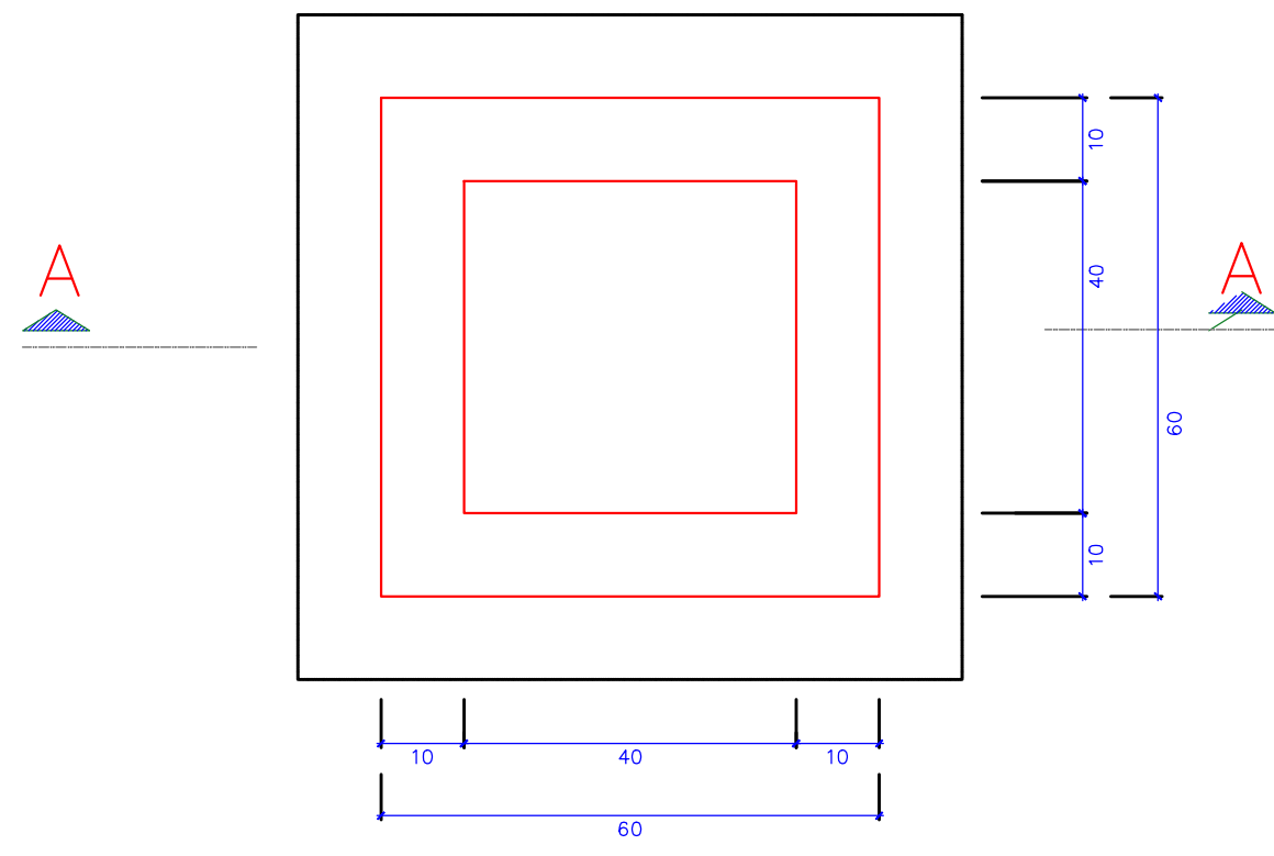
PLANTA BAIXA CAIXA DE PASSAGEM CP ESCALA - 1 : 10
