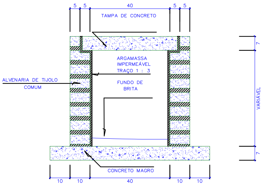
CORTE A.A. ESG. 1 : 10
