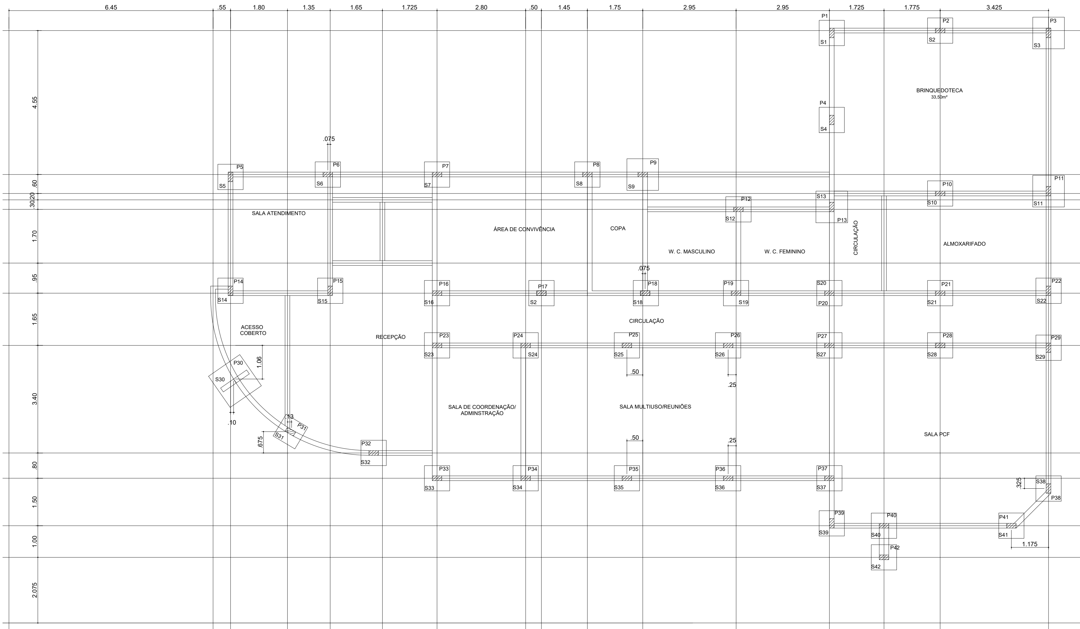
PLANTA DE LOCAÇÃO SAPATAS ESCALA: 1 / 50
