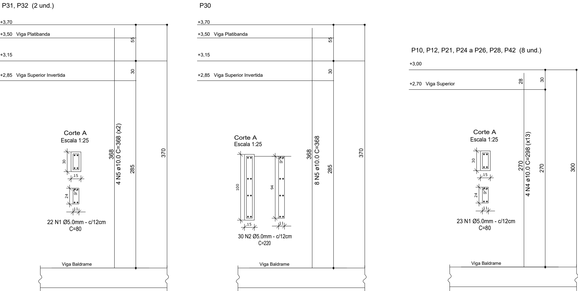
RESUMO DO AÇO PILARES
