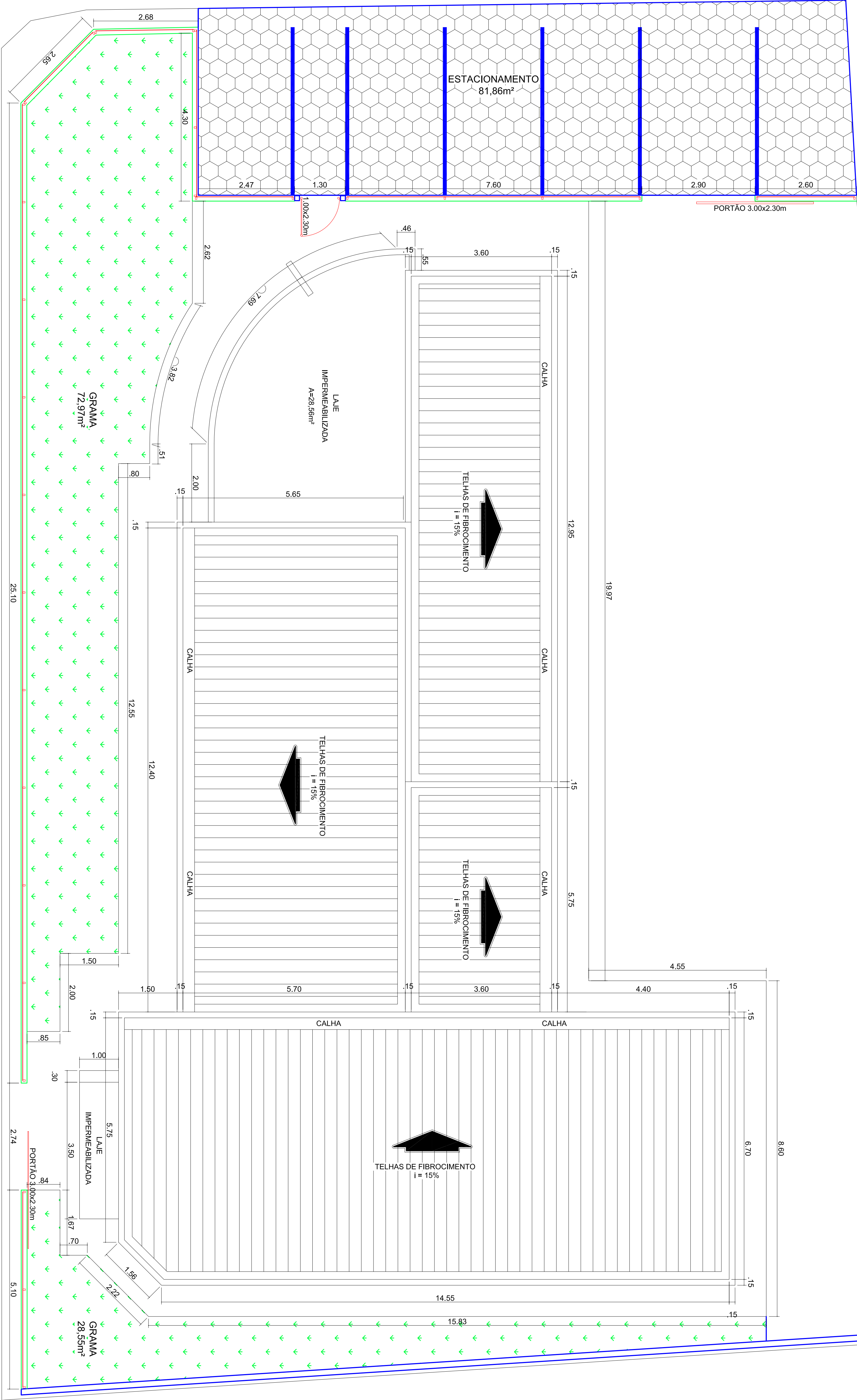
PLANTA DE LOCAÇÃO/COBERTURA ESCALA: 1 / 75
